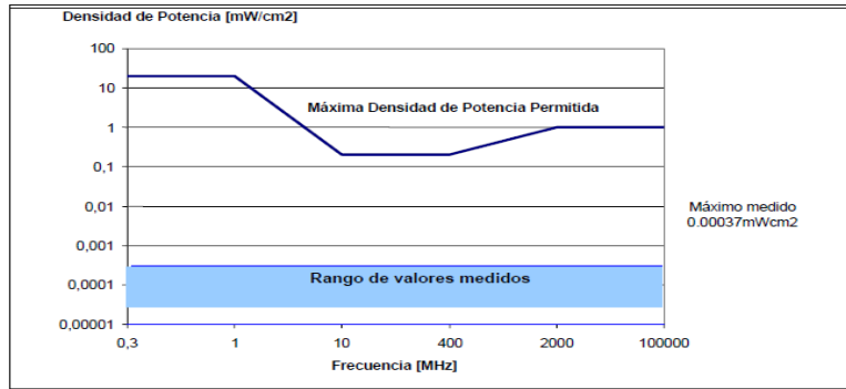
Gráfico 1: Máximos admisibles de densidad de potencia permitidos y Rangos de valores medidos
